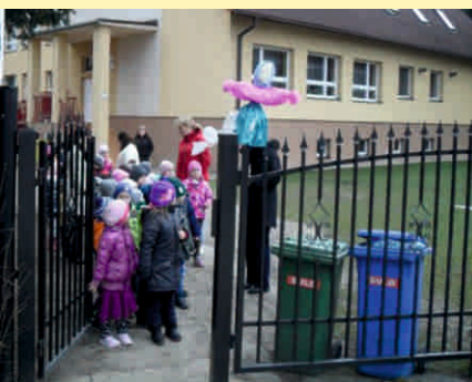
Vynášanie moreny
